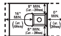
NON-COMBUSTIBLE FLOOR PROTECTOR PROTÉCTEUR DE PLANCHER INCOMBUSTIBLE
